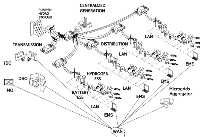
Figura 1. Estructura de microrredes cooperativas
