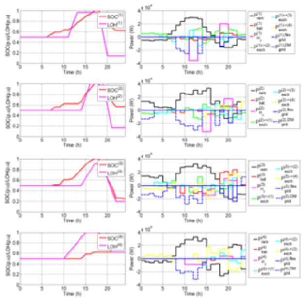
Figura 9. Servicios de flexibilidad Bext= 170 euros.
